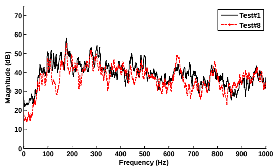
شکل ۱۴- حوزه فرکانسی سیگنال ذخیره شده آزمایش‌های اول و هشتم (فاصله ۵۰ سانتی‌متری از سمت BC).
