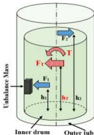
شکل ۱- دیاگرام آزاد یک ماشین لباسشویی عمودی.
