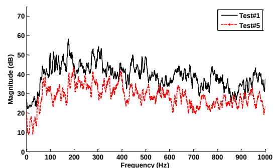
شکل ۱۱- حوزه فرکانسی سیگنال ذخیره شده آزمایش‌های اول و پنجم (فاصله ۵۰ سانتی‌متری از سمت BC).
