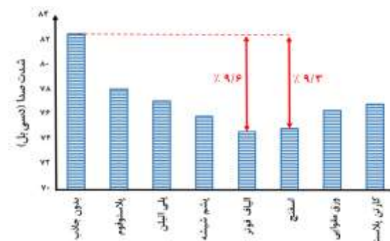
شکل ۳- شدت صدا در فاصله ۵۰ سانتی متری
