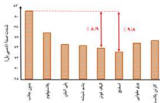
شکل ۴- شدت صدا در فاصله ۱۰۰ سانتی متری
