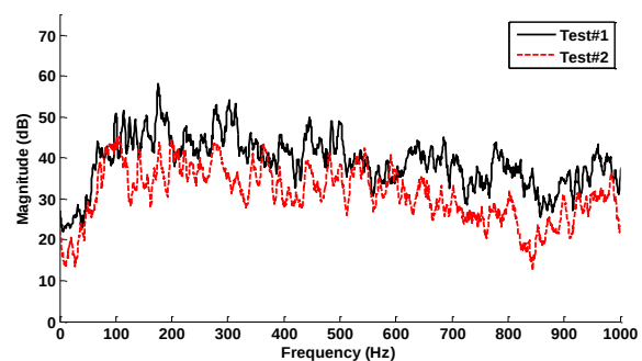
شکل ۸- حوزه فرکانسی سیگنال ذخیره شده آزمایش‌های اول و دوم (فاصله ۵۰ سانتی‌متری از سمت BC).
