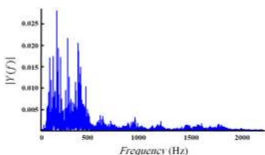
شکل ۷- سیگنال حوزه فرکانس ذخیره شده آزمایش اول، فاصله ۱۰۰ سانتی متری از لباسشویی
