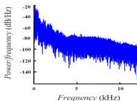
شکل ۶- نمودار طیف سیگنال آزمایش اول، فاصله ۱۰۰ سانتی متری از ماشین لباسشویی
