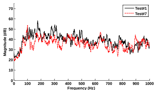
شکل ۱۳- حوزه فرکانسی سیگنال ذخیره شده آزمایش‌های اول و هفتم (فاصله ۵۰ سانتی‌متری از سمت BC).
