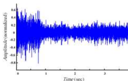
شکل ۵- سیگنال حوزه زمان ذخیره شده مربوط به آزمایش اول، فاصله ۱۰۰ سانتی متری از ماشین لباسشویی
