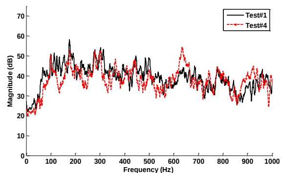
شکل ۱۰- حوزه فرکانسی سیگنال ذخیره شده آزمایش‌های اول و چهارم (فاصله ۵۰ سانتی‌متری از سمت BC).
