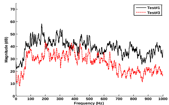
شکل ۹- حوزه فرکانسی سیگنال ذخیره شده آزمایش‌های اول و سوم (فاصله ۵۰ سانتی‌متری از سمت BC).
