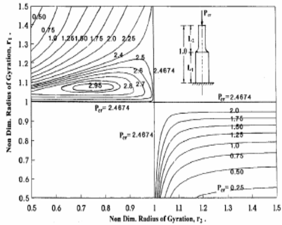
شکل ۳- تغییر بار بحرانی بهینه بر حسب شعاع های ژیراسیون برای یک ستون دو تکه و با مقطع توپر
