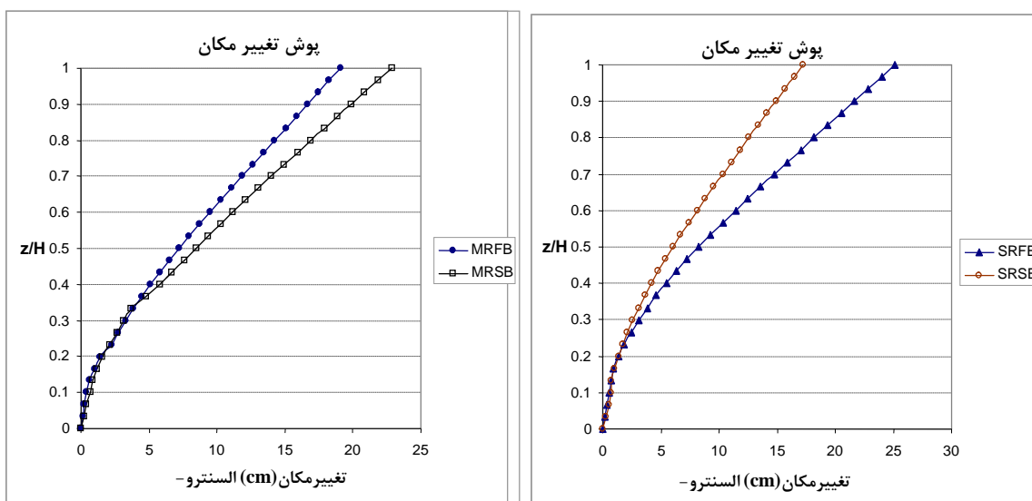
الف. پوش تغییر شکل برای مدل های با مخزن المان محدود ب. پوش تغییر شکل برای مدل های با مخزن جرم افزوده شکل ۱۳- اثرات مدل سازی سنگ پی بر پوش تغییر شکل - زلزله السنترو
