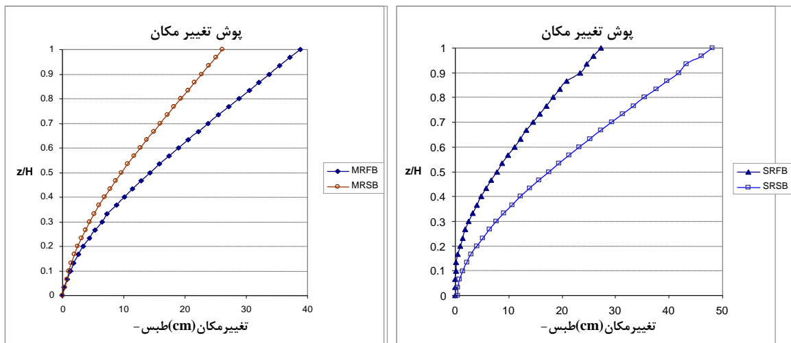
الف. پوش تغییر شکل برای مدل های با مخزن المان محدود ب. پوش تغییر شکل برای مدل های با مخزن جرم افزوده شکل ۱۱- اثرات مدل سازی سنگ پی بر پوش تغییر شکل - زلزله طبس
