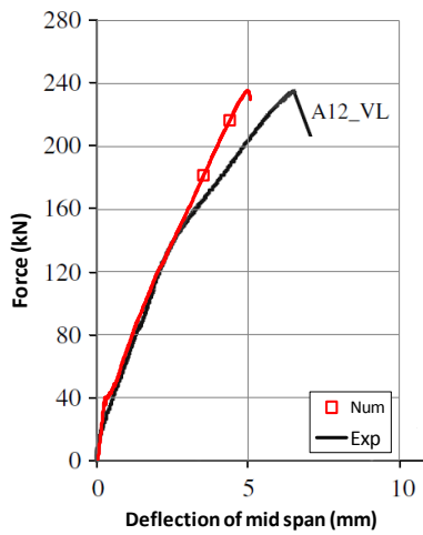
شکل ۸- منحنی نیرو-تغییر مکان تیرهای گروه اول - نتایج مدل‌های عددی در مقایسه با نتایج آزمایشگاهی
