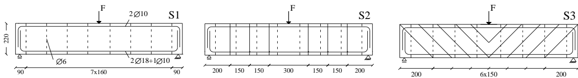
شکل ۲- نمونه‌های در نظر گرفته شده برای مدل‌سازی عددی - گروه دوم
