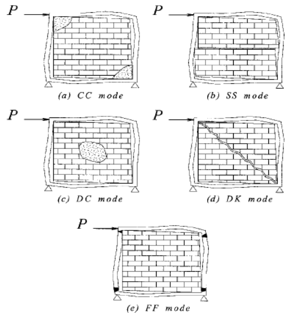
شکل ۱- مدهای مختلف خرابی قاب‌های میانپیر با مصالح بنایی (a) مد خرد شدگی کنج، (b) مد برش لغزشی، (c) مد فشار قطری، (d) مد ترک قطری، (e) مد شکست قاب [V]
