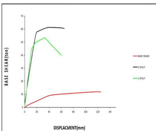
شکل ۹- نمودار برش پایه-تغییرمکان قاب دو طبقه با میانقاب ۳۵cm
