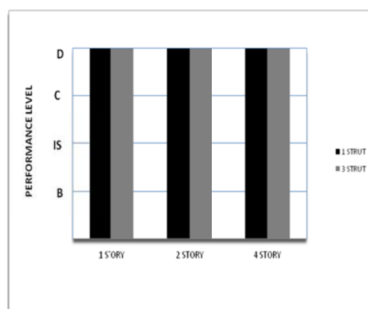
شکل ۱۶- نمودار سطوح عملکرد دستک‌ها در قاب با میانقاب ۳۵cm
