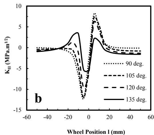
شکل ۱۳- روند تغییرات K_{II} به ازای زوایای مختلف استقرار ترک (a) ۴۵-۹۰ درجه و (b) ۹۰-۱۳۵ درجه
