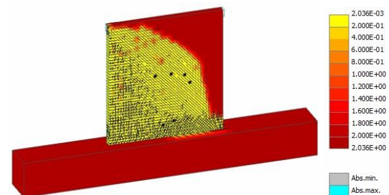
شکل ۳۱- توزیع مقاومت کششی و ترک نهایی برای S=15\text{cm}
