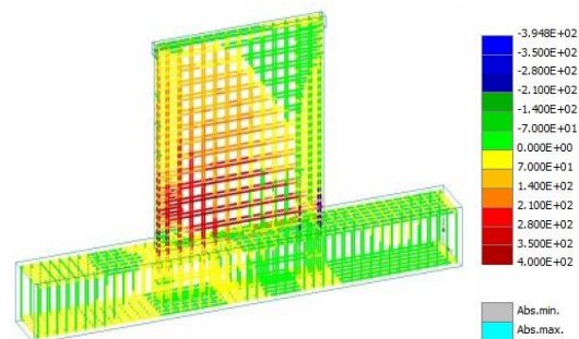
شکل ۱۷- توزیع تنش نهایی در میلگرد
