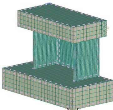
شکل ۵- مش بندی مدل تحلیلی و محل اعمال بار و اندازه‌گیری تغییر مکان جانبی
