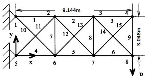
شکل ۶- طرح اولیه خرپا ۱۵ لینیکی
