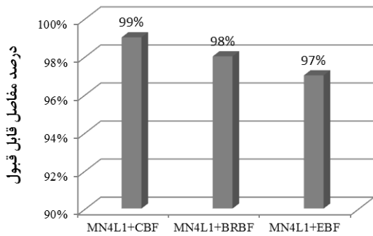
الف- درصد مفاصل قابل قبول نمونه ۴ طبقه
