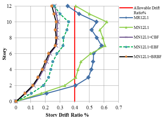
ج- مقدار تغییر مکان نسبی طبقات نمونه ۱۲ طبقه
