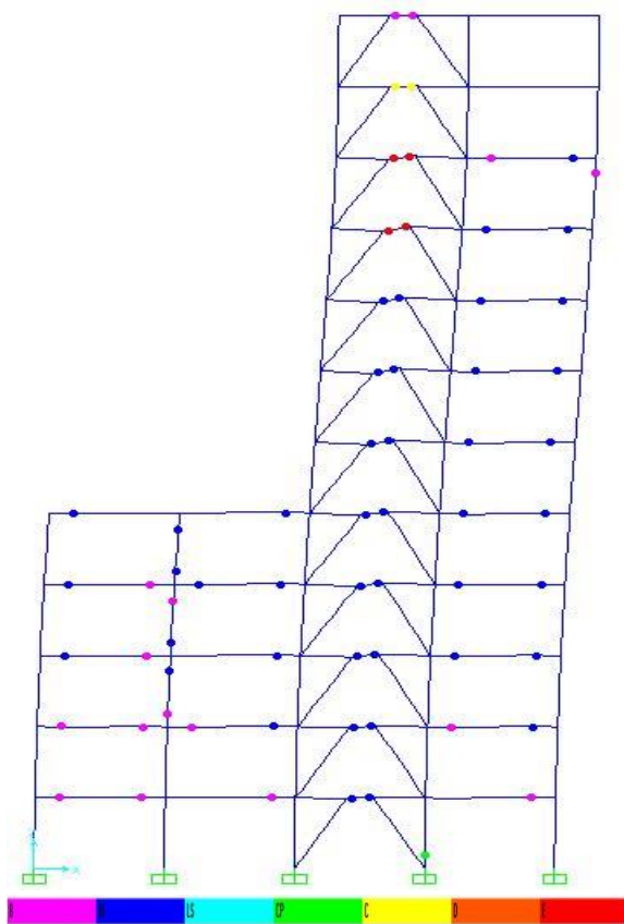
الف- نمونه MN^{۱۲}L^{۱}+EBF
