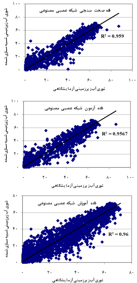
شکل ۲: شوری آب زیرزمینی زیر لوله‌های زهکش در مراحل مختلف فعالیت شبکه عصبی و مقادیر آزمایشگاهی (دسی زیمنس بر متر)
