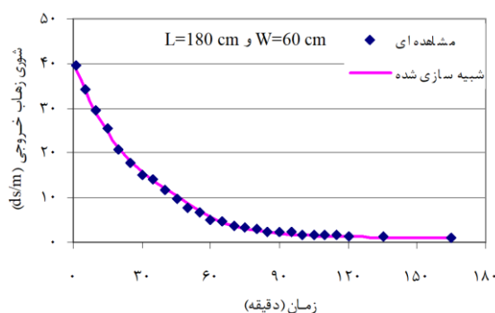
شکل ۴: شبیه‌سازی تغییرات شوری خروجی از زهکش‌ها با دبی ثابت 0/14 لیتر بر ثانیه نسبت به زمان
