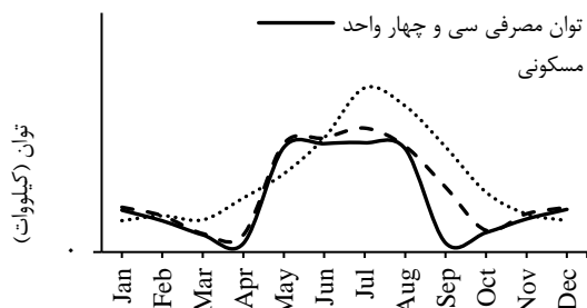
شکل ۱۴- سیستم هیبریدی توربین باد و پیل سوختی برای سی و چهار واحد مسکونی در زابل
