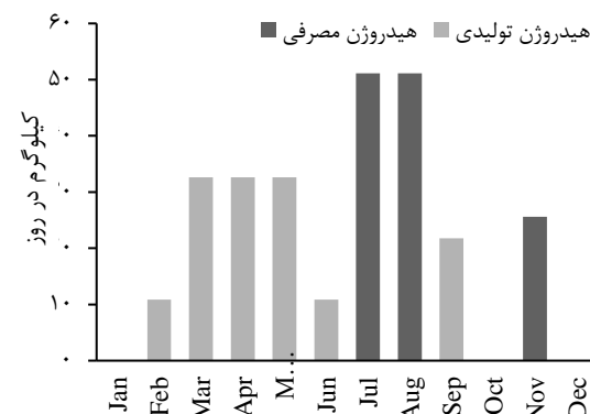
شکل ۹- مقایسه هیدروژن تولیدی و مصرفی سیستم هیبریدی برای شش واحد مسکونی در تهران
