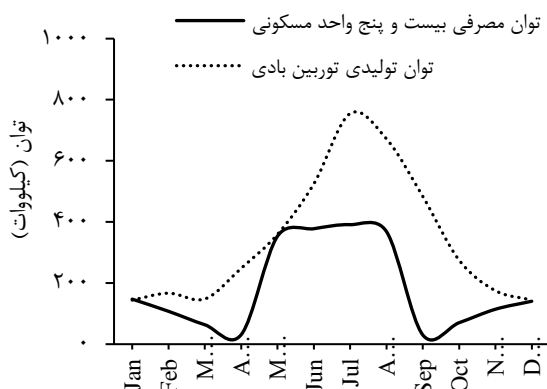
شکل ۱۳- مقایسه توان مصرفی ۲۵ واحد مسکونی و توان تولیدی یک توربین بادی ۸۵۰ کیلوواتی برای شهر زابل
