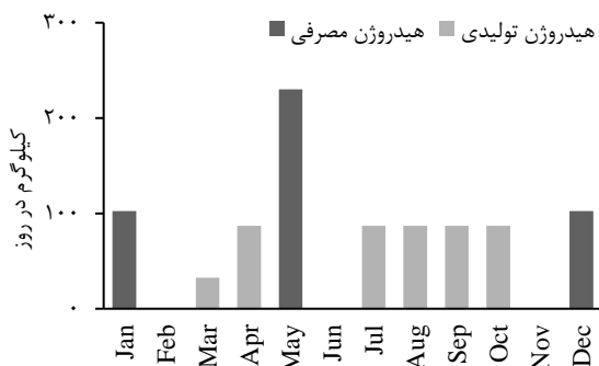
شکل ۱۵- مقایسه هیدروژن تولیدی و مصرفی سیستم هیبریدی برای سی و چهار واحد مسکونی در زابل
