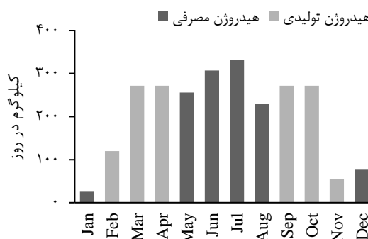
شکل ۱۲- مقایسه هیدروژن تولیدی و مصرفی سیستم هیبریدی برای شصت و هشت واحد مسکونی در منجیل
