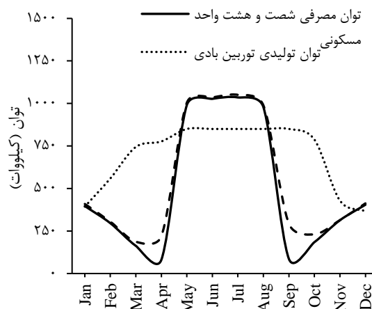
شکل ۱۱- سیستم هیبریدی توربین باد و پیل سوختی برای شصت و هشت واحد مسکونی در منجیل
