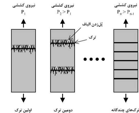
شکل ۲: نحوه تشکیل ترک‌های چندگانه در مصالح HPFRCC [۶]
