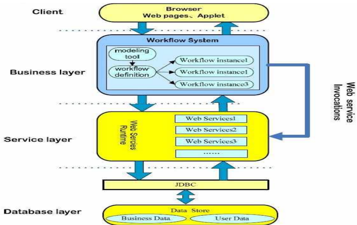
شکل ۱- معماری سازنده کد Shan و همکاران
