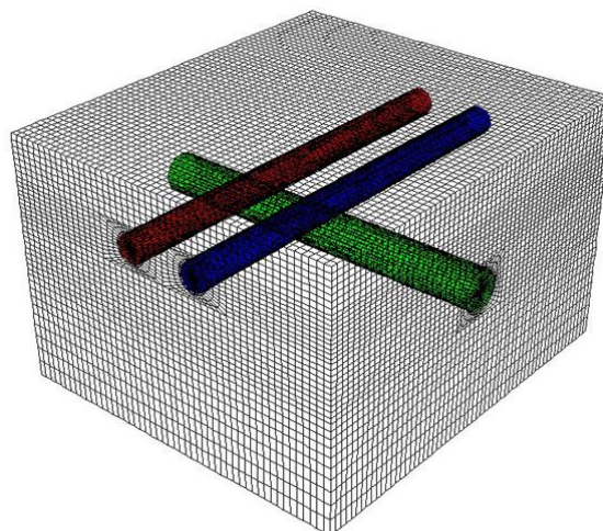
شکل ۶: مدل ایجاد شده برای تقاطع غیر همسطح خطوط ۲ و ۳ مترو تبریز
