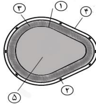
۱- هسته و المنت ۲- ترموکوپل ۳- ماسه بادی ۴- سطح لوله بادامک شکل (مسی) عایق ۵- عایق الف- شماتیک لوله برای اندازه‌گیری دمای سطح
