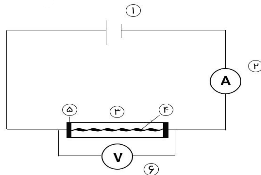
۱- دیمتر صنعتی ۲- آمپر متر ۳- لوله تحت آزمایش ۴- هسته و المنت ۵- عایق ۶- ولت‌متر شکل ۵- مدار الکتریکی آزمایش
