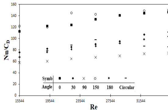
شکل ۱۲- تغییرات عملکرد هیدرولیکی- حرارتی لوله بادامکی شکل بر حسب عدد رینولدز در زوایای حمله متفاوت در شار حرارتی ۳۲۶۹ W/m 2
