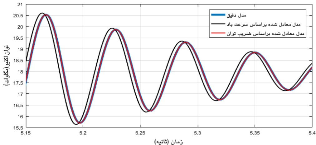
شکل ۱۴-ب: نمایی نزدیک از توان اکتیو در هنگام افت ولتاژ
