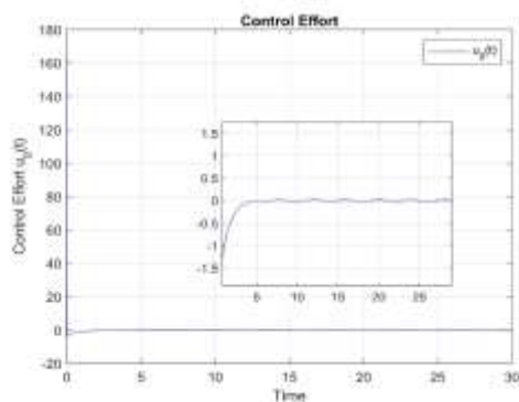
شکل ۲۰.۲ - ورودی کنترلی u_0(t)
