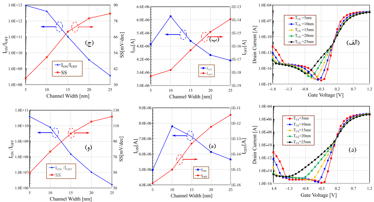
شکل ۴- جریان درین به صورت تابعی از ولتاژ گیت به ازای ضخامت‌های مختلف کانال ( T_{ch} ) و (الف) ولتاژ درین ۰/۱ ولت و (د) ولتاژ درین ۰/۵ ولت. جریان روشنایی و جریان خاموشی برای (ب) ولتاژ درین ۰/۱ ولت و (ه) ولتاژ درین ۰/۵ ولت. قابل توجه است که محور جریان روشنایی خطی و جریان خاموشی به صورت لگاریتمی است. نسبت جریان روشنایی به جریان خاموشی و پش زیرآستانه برای (ج) ولتاژ درین ۰/۱ ولت و (و) ولتاژ درین ۰/۵ ولت.
