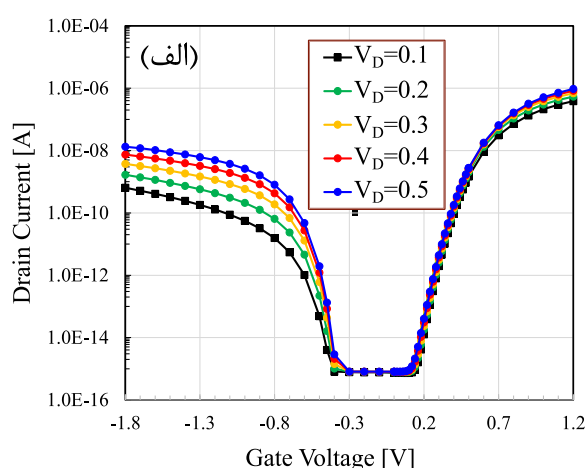
شکل ۲ - جریان درین به صورت تابعی از ولتاژ گیت برای ترانزیستور تونل زنی عمودی مبتنی بر (الف) ژرمانیوم و (ب) گالیوم-آرسناید.
