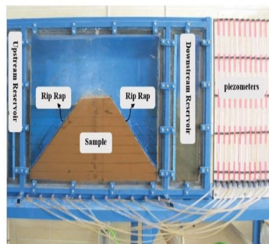
شکل ۳- فلوم مورد بررسی در مدل آزمایشگاهی [۲۶].
