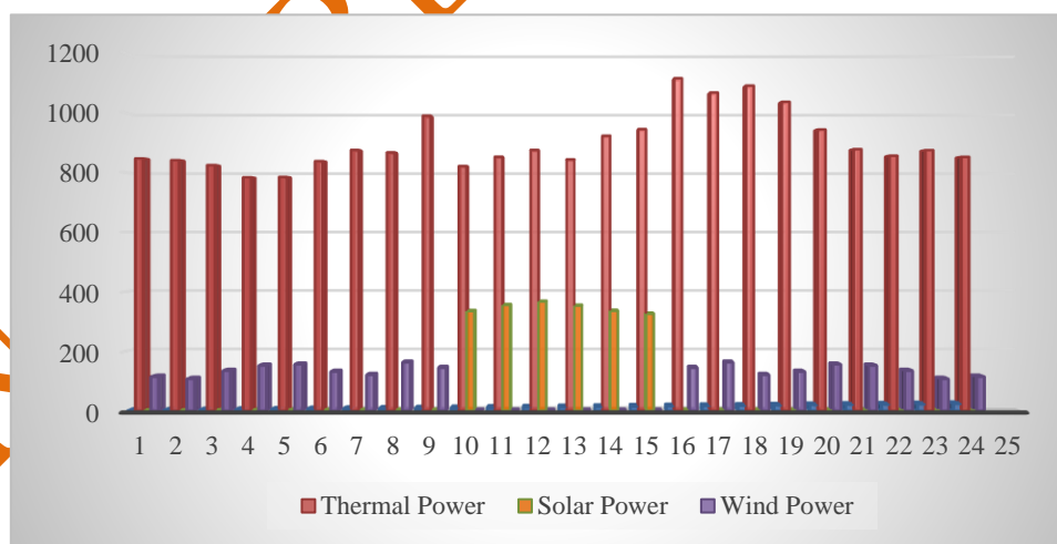
شکل ۱ سهم واحدهای تولیدی مختلف در طول یک شبانه روز
