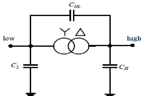
شکل (۷): مدل فرکانس بالای ترانسفورماتور [۱۴]
