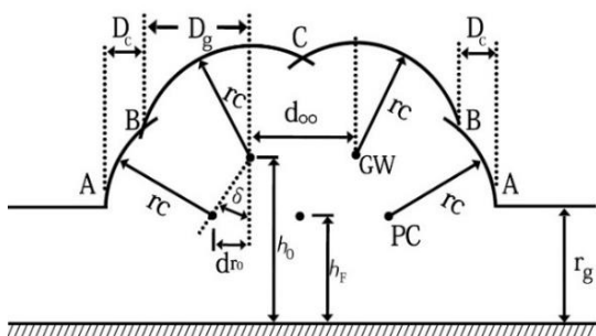
شکل (۹): مدل EGM ترسیم شده با توجه به محل قرارگیری سیم‌های محافظ و هادی‌های فاز
