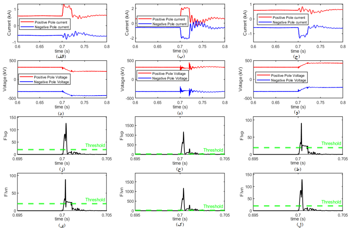
شکل ۶- عملکرد طرح حفاظتی به ازای خطای داخلی PG, PN, و NG (الف)-(ج) جریان قطب مثبت و منفی (د)-(و) ولتاژ قطب مثبت و منفی (ز)-(ط) شاخص انرژی قطب مثبت. (ی)-(ل) شاخص انرژی قطب منفی
