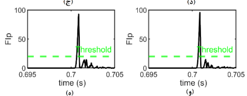
شکل ۱۲- بررسی اثر مقدار راکتور بر عملکرد طرح
