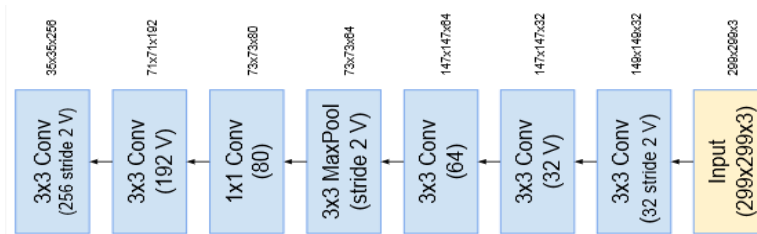
شکل ۳: معماری مدل Inception-ResNet-V2
