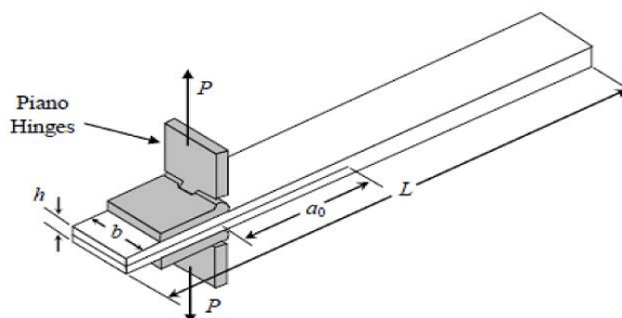
شکل ۱- شکل شماتیک چیدمان تست تیر گیردار دولبه برای اندازه‌گیری چقرمگی شکست مربوط به مود اول [۱۹].
