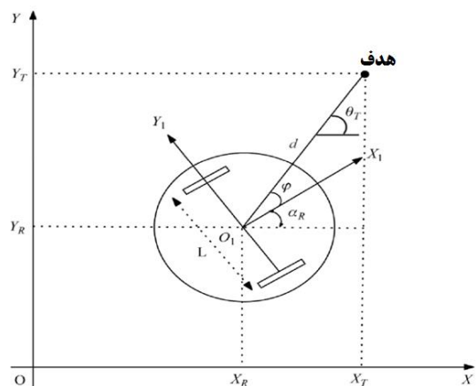
شکل ۳- زاویه بین ربات و هدف.
