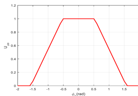
شکل ۸- تابع سودمندی عامل اجتناب از مانع وابسته به زاویه
