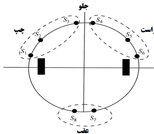
شکل ۴- موقعیت هشت سنسور بر روی ربات
