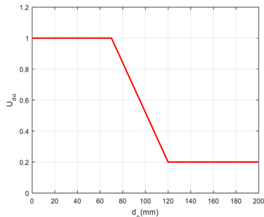
شکل ۷- تابع سودمندی عامل اجتناب از مانع وابسته به فاصله
