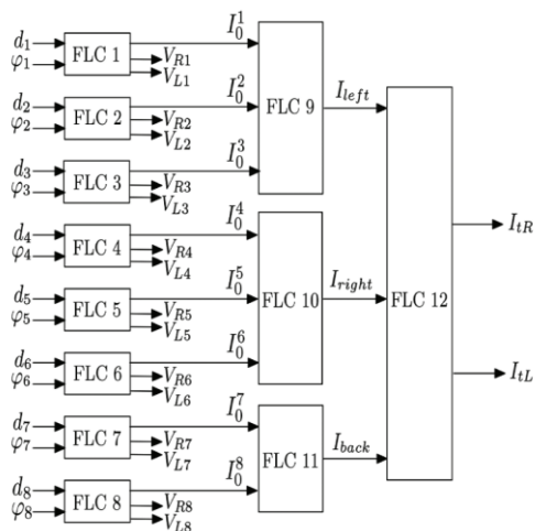
شکل ۵- بلوک دیاگرام سیستم فازی سلسله مراتبی
