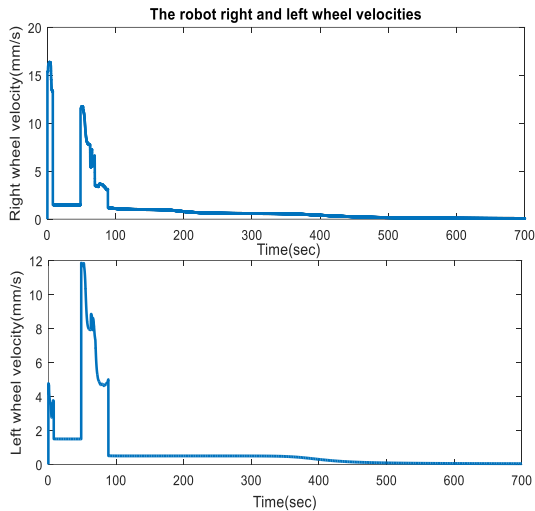
شکل ۱۲: سرعت چرخ راست و چپ ربات در حضور دو مانع
