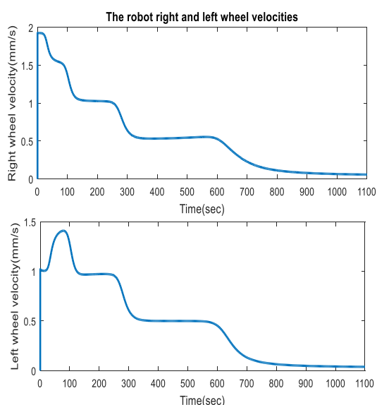
شکل ۱۰- سرعت چرخ راست و چپ ربات
