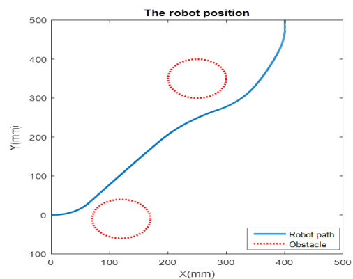
شکل ۱۴: مسیر طی شده توسط مرکز ربات در حضور دو مانع
