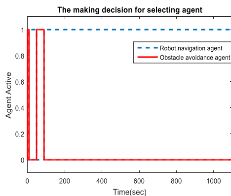
شکل ۱۳: نحوی فعال شدن عوامل ناوبری ربات و اجتناب از مانع در حضور دو مانع
