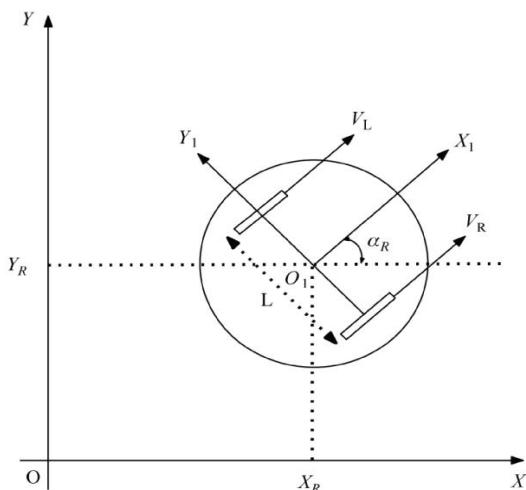
شکل ۱- مدل شماتیکی از ربات سیار
