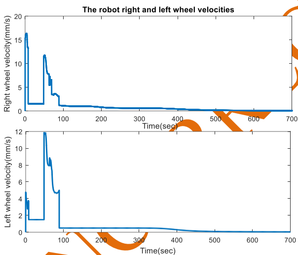
شکل ۱۳: سرعت چرخ راست و چپ ربات در حضور دو مانع
