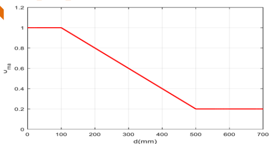
شکل ۶- تابع کاربردی عامل ناوبری ربات
