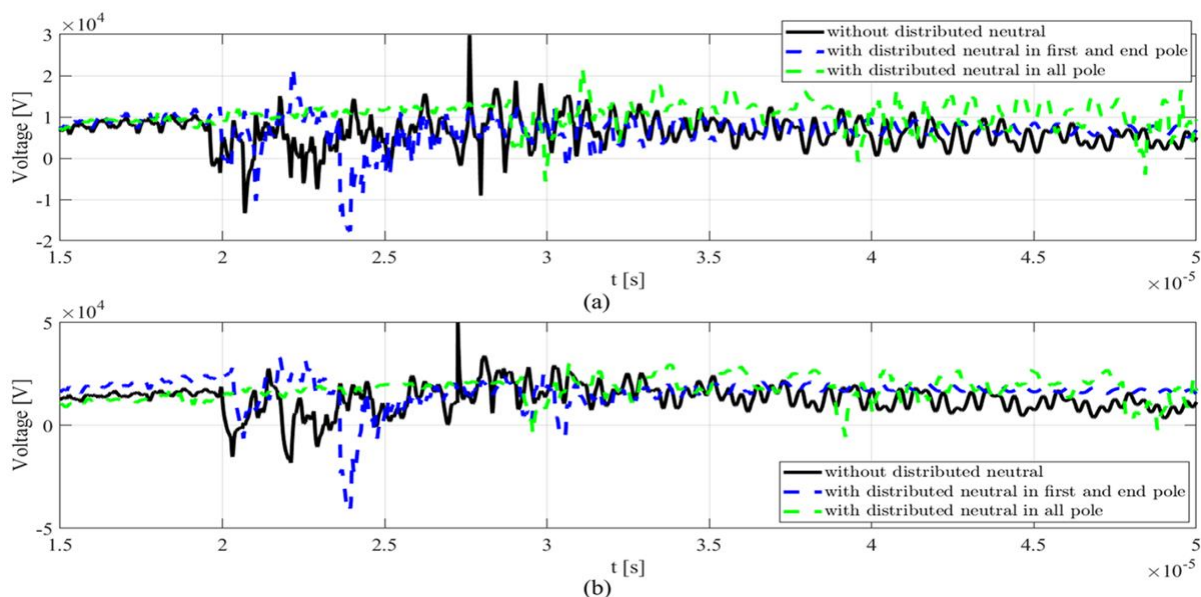
شکل ۱۷- ولتاژ در ترمینال مصرف‌کنندگان ابتدا و انتهای فیدر دو، با نصب SPD در سمت فشار ضعیف ترانسفورماتور، در حالات بدون زمین کردن نول و زمین کردن نول در پایه‌های ابتدا و انتهای فیدرها و همی پایه‌های هر دو فیدر؛ (a) بار شماره ۶ (b) بار شماره ۸
