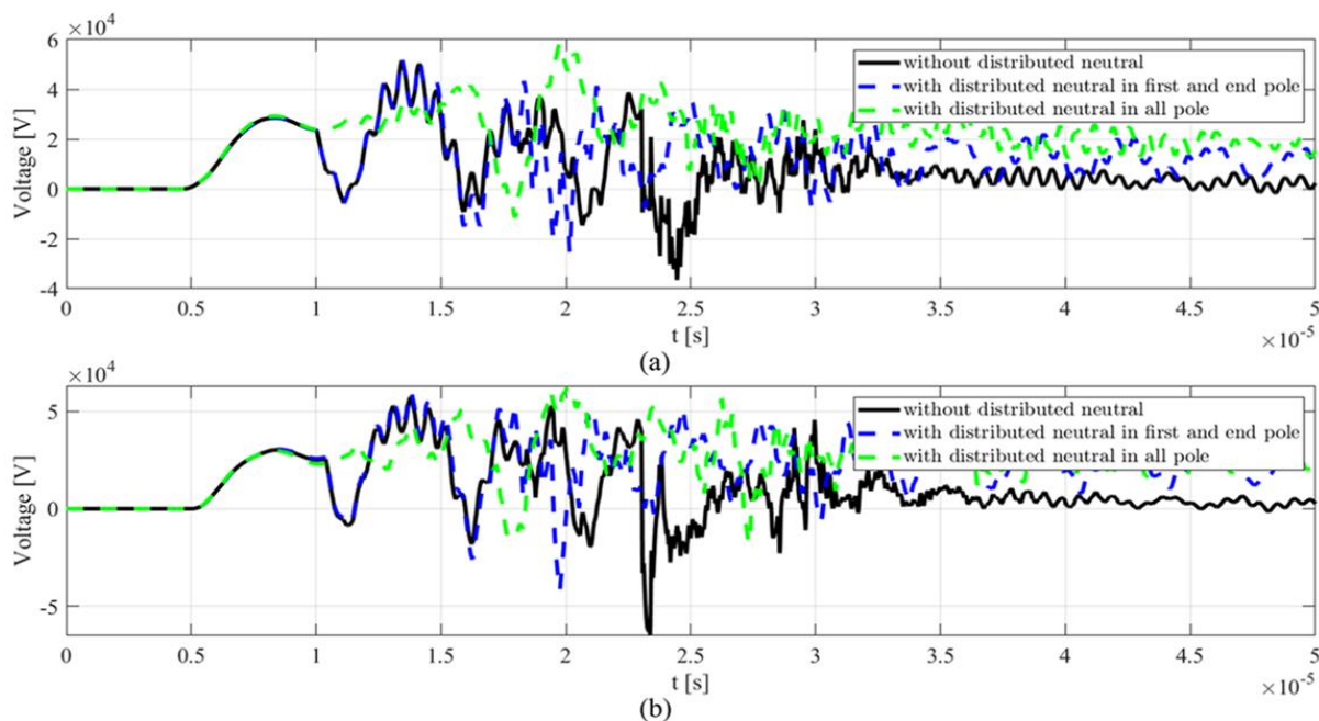
شکل ۱۶- ولتاژ در ترمینال مصرف‌کنندگان ابتدا و انتهای فیدر دو، بدون نصب SPD در سمت فشار ضعیف ترانسفورماتور، در حالات بدون زمین کردن نول و زمین کردن نول در پایه‌های ابتدا و انتهای فیدرها و همی پایه‌های هر دو فیدر؛ (a) بار شماره ۶ (b) بار شماره ۸
