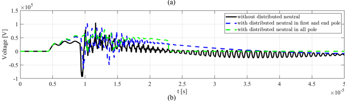
شکل ۱۵- ولتاژ در ترمینال مصرف‌کنندگان ابتدا و انتهای فیدر یک، با نصب SPD در سمت فشارضعیف ترانسفورماتور، در حالات بدون زمین کردن نول و زمین کردن نول در پایه‌های ابتدا و انتهای فیدرها و هم‌هی پایه‌های هر دو فیدر؛ (a) بار شماره ۱ (b) بار شماره ۵
