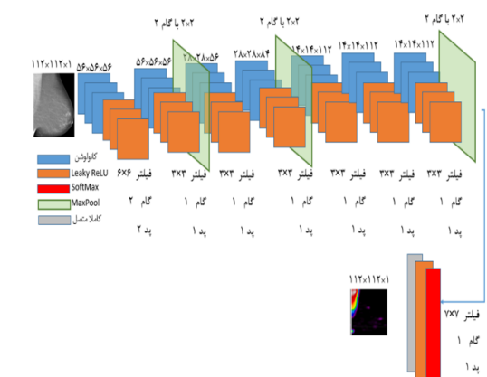
شکل ۴. معماری شبکه عصبی کانولوشنی عمیق پیشنهادی (DCNN)
