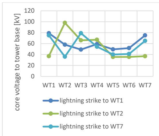
شکل ۲۷- اضافه‌ولتاژها در مزرعه بادی موازی با پیوند ضربدری و سیستم زمین یکپارچه
