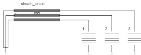
الف) نحوه اجرای پیوند تک نقطه‌ای
