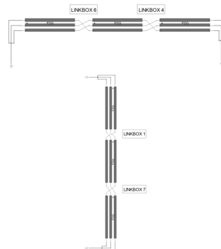
شکل ۱۵- اجرای پیوند ضربدری در آرایش موازی توربین‌ها
