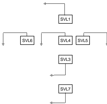
ب) آرایش نصب محدودسازهای ولتاژ غلاف در مزرعه بادی موازی با پیوند تک نقطه‌ای
