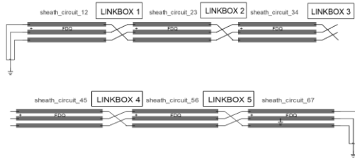
شکل ۱۸- پیوند ضربدیری در مزرعه بادی سری با SVL
