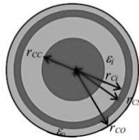
شکل ۷- سطح مقطع کابل استفاده شده در مزرعه بادی
