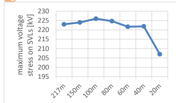
شکل ۲۶- بیشینه تنش ولتاژی در محدودسازهای ولتاژ غلاف مزرعه بادی سری با پیوند تک‌نقطه‌ای به ازای فواصل مختلف بین توربین‌ها
