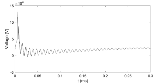
شکل ۱۰- شکل موج بیشترین اضافه‌ولتاژ ایجاد شده در مزرعه بادی موازی با پیوند تک‌نقطه‌ای ناشی از اصابت صاعقه به
