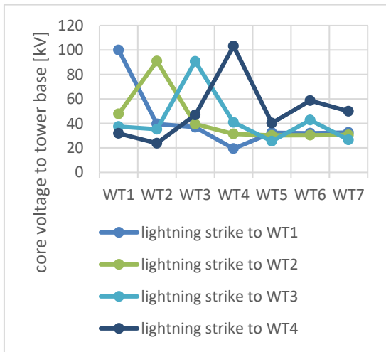
شکل ۱۲- اضافه‌ولتاژهای ایجاد شده در نقاط مختلف شبکه کابلی مزرعه بادی سری با پیوند تک‌نقطه‌ای
