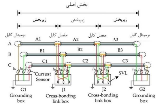
شکل ۱۴- نمایش اجرای پیوند ضربدری در یک کابل [۲۹]
