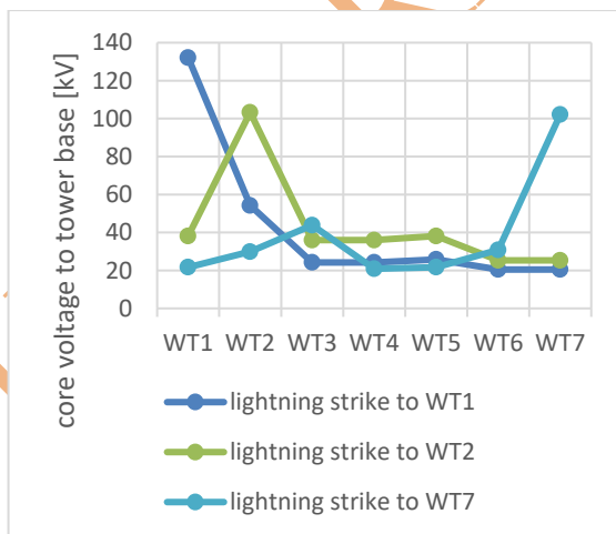
شکل ۹- توزیع اضافه‌ولتاژها در شبکه کابلی مزرعه بادی موازی با پیوند تک نقطه‌ای
