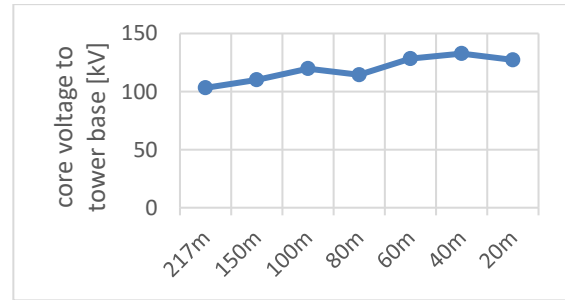
شکل ۲۴- تنش‌های ولتاژی در شبکه کابلی مزرعه بادی سری با پیوند تک‌نقطه‌ای به ازای کاهش فاصله بین توربین‌ها
