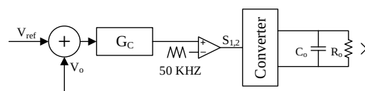
شکل ۱۸- بلوک دیاگرام سیستم کنترل برای مبدل پیشنهادی
