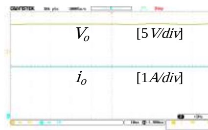
شکل ۲۴- نتایج آزمایشگاهی: ولتاژ/جریان خروجی در حالت کاهنده
