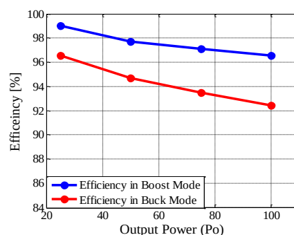
شکل ۹- بازده بر حسب توان خروجی (حالت‌های افزایشده و کاهشده)
