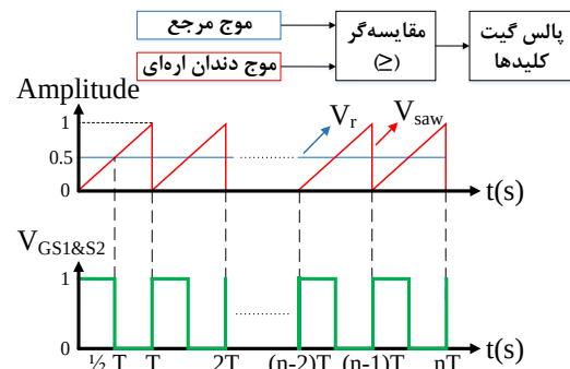
شکل ۴- نحوه تولید پالس‌های گیت سوئیچ‌های مبدل
