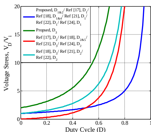
شکل ۱۴- مقایسه تنش ولتاژ دیودها
