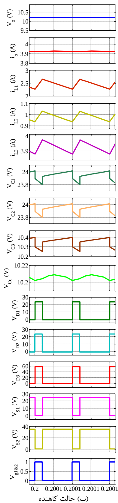
شکل ۱۹- شکل موج‌های نتایج شبیه‌سازی مبدل پیشنهادی در دو حالت افزایشی و کاهنده
