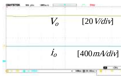
شکل ۲۳- نتایج آزمایشگاهی: ولتاژ/جریان خروجی در حالت افزایشده
