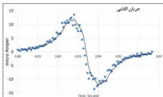
شکل ۴- نمودار جریان القاء شده به الکتروده
