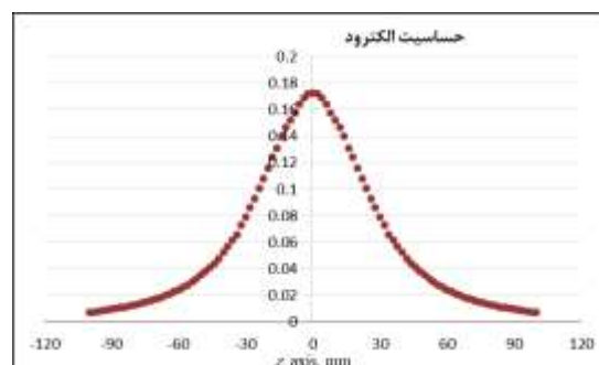
شکل ۳- نمودار حساسیت الکتروده در طول \pm 100 میلی‌متر از محور Z در هر ۲ میلی‌متر
