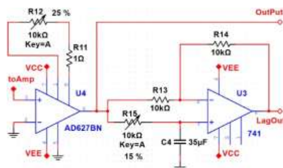
شکل ۸- تقویت کننده ابزار دقیق با مدار تصحیح فاز
