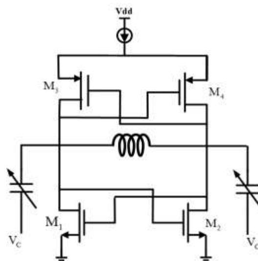
شکل ۹- مدار VCO
