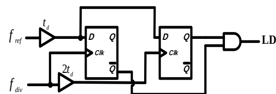
شکل ۴- آشکارساز قفل
