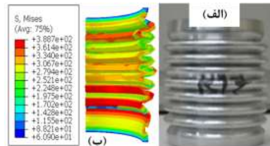
شکل ۶- لوله پس از لهیدگی: (الف) تجربی [۱۰]، (ب) شبیه‌سازی
