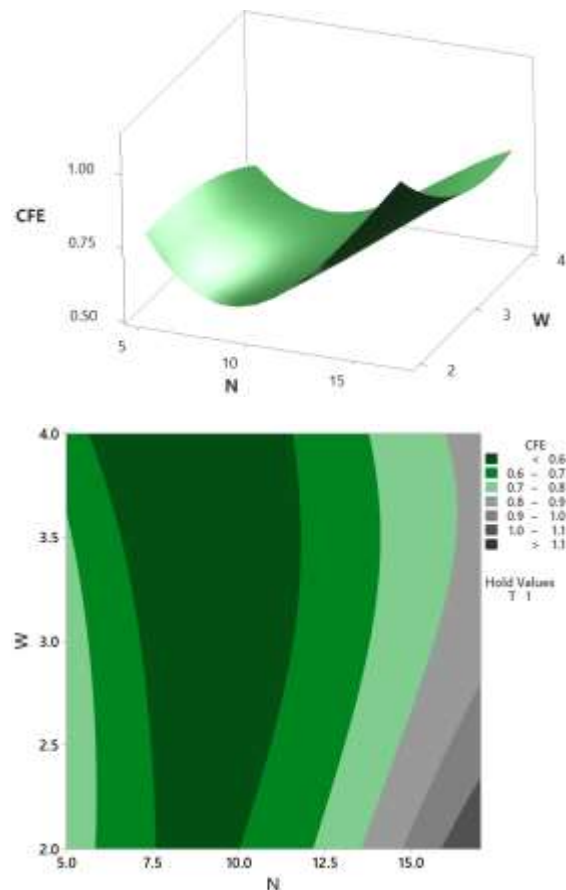
شکل ۱۲- رویه سه‌بعدی و کانتوری دوبعدی بازده نیروی لهدیگی بر حسب تعداد و عرض شیار
