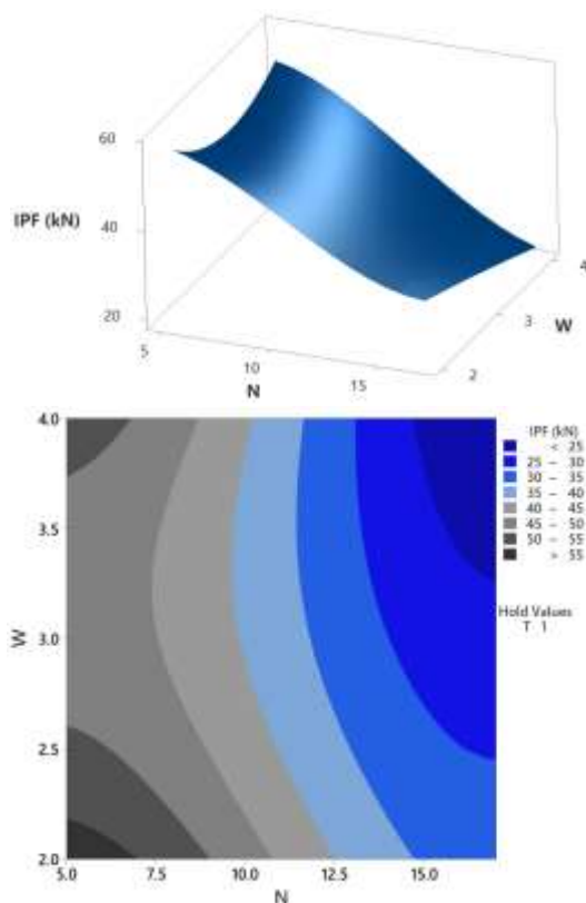
شکل ۸- رویه سه‌بعدی و کانتوری دوبعدی نیروی لهیدگی اولیه بر حسب تعداد و عرض شیار
