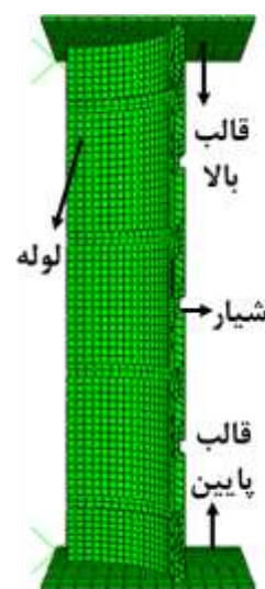
شکل ۳- مدل اجزای محدود طراحی شده
