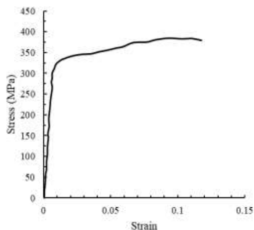
شکل ۱- نمودار تنش-کرنش حقیقی آلومینیوم پیرسخت شده
