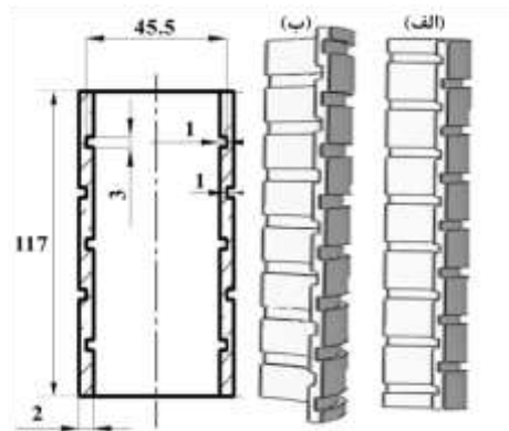
شکل ۵- الگوی شیپرها: الف) نوع ۱، ب) نوع ۲
