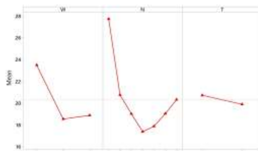
شکل ۹- تاثیر پارامترهای ورودی بر روی جذب انرژی مخصوص
