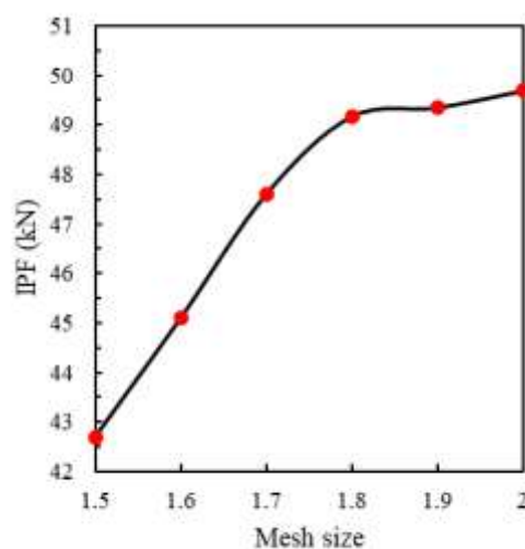
شکل ۲- همگرایی سائز المان
