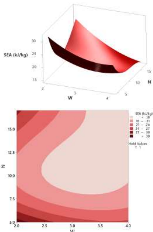
شکل ۱۰- رویه سه بعدی و کانتوری دوبعدی جذب انرژی مخصوص بر حسب عرض و تعداد شیار
