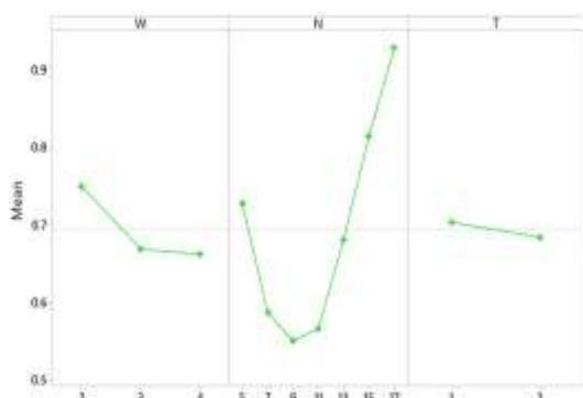
شکل ۱۱- تاثیر پارامترهای ورودی بر روی بازده نیروی لهیدگی
