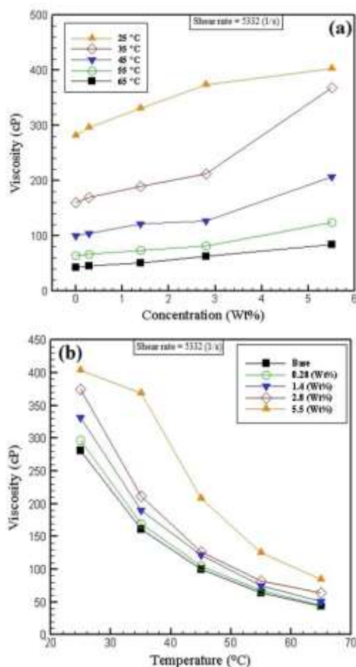
شکل ۳- (a) ویسکوزیته بر حسب غلظت در دماهای تحت آزمایش. (b) ویسکوزیته بر حسب دما در غلظت های مختلف
