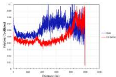
شکل ۷- ضریب اصطکاک نسبت به مسافت در دمای ۲۰۰ درجه سانتی گراد برای روغن پایه خالص و نانوسیال با غلظت ۲/۸ درصد وزنی.
