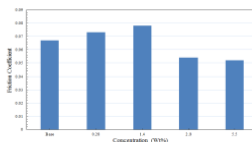
شکل ۵- ضریب اصطکاک در غلظت‌های مختلف در دمای محیط
