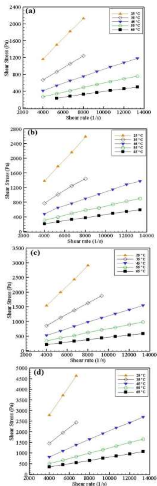
شکل ۲- نمودار تنش برشی بر حسب نرخ برش در دماهای مختلف برای غلظت (a) ۰/۲۸ درصد وزنی (b) ۱/۴ درصد وزنی (c) ۲/۸ درصد وزنی (d) ۵/۵ درصد وزنی
