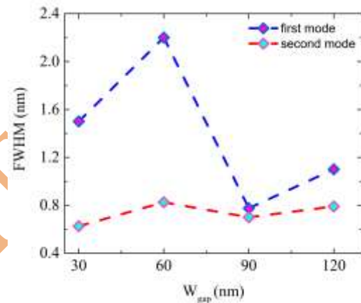
شکل ۴- (الف) رابطه طیف خاموشی و (ب) پهنای کامل در نصف مقدار توان بیشینه برای فاصله گپ‌های مختلف.
