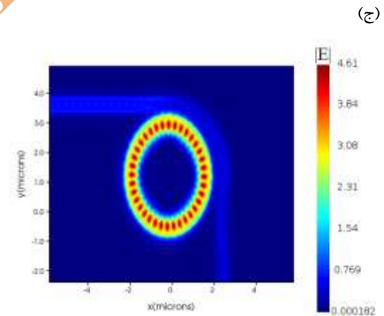
شکل ۶- (الف) طیف انتقال نرمالیزه شده برای تشدیدگر میکرو دیسکی با موجبر خمیده ۹۰ درجه بر حسب طول موج. نمایه میدان الکتریکی (ب) مد اول و (ج) مد دوم.
