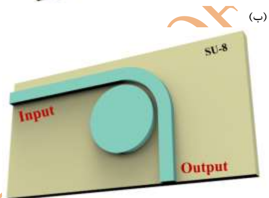
شکل ۱- ساختار حسگر میکرو دیسکی با موجبر خمیده (الف) ۱۸۰ درجه و (ب) ۹۰ درجه.
