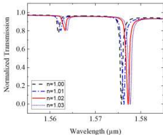
شکل ۵- نمودار تغییرات طیف انتقال به هنگام تغییر ضریب شکست محیط اطراف حسگر با موجبری با انحنای ۱۸۰ درجه.
