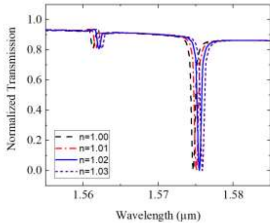
شکل ۷- نمودار تغییرات طیف انتقال به هنگام تغییر ضریب شکست محیط اطراف حسگر با موجبری با انحنای ۹۰ درجه.
