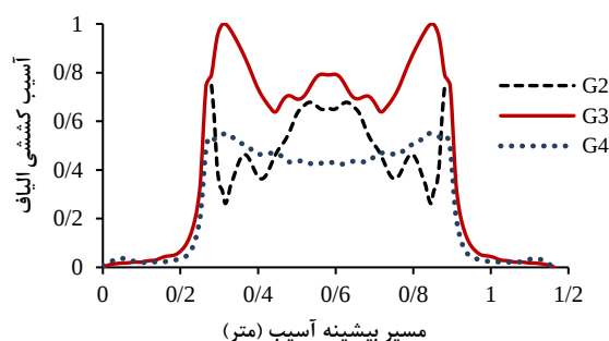
شکل ۱۴- آسیب کششی وارده به الیاف براساس معیار هاشین
