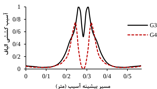
شکل ۲۱- آسیب کششی وارده به الیاف براساس معیار هاشین
