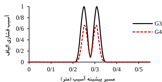
شکل ۲۰- آسیب فشاری وارده به الیاف براساس معیار هاشین
