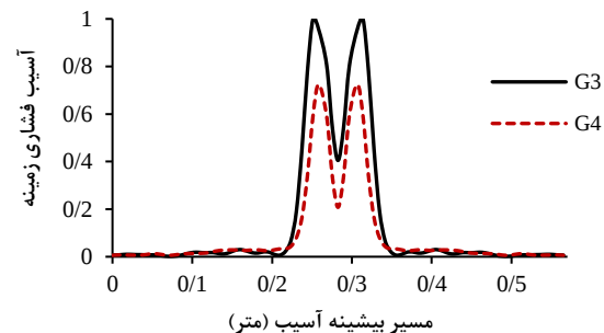
شکل ۲۲- آسیب فشاری وارده به زمینه براساس معیار هاشین
