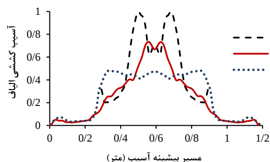
شکل ۷- آسیب کششی وارده به الیاف براساس معیار هاشین
