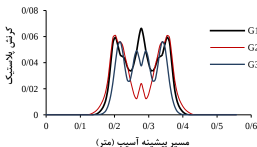
شکل ۱۸- کرنش پلاستیک معادل در مسیر بیشینه آسیب
