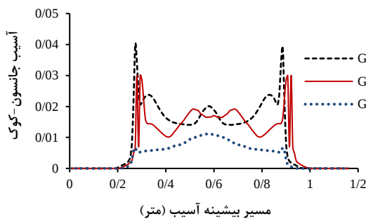
شکل ۵- آسیب وارده به مخازن براساس معیار جانسون-کوک
