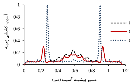
شکل ۱۶- آسیب کششی وارده به زمینه براساس معیار هاشین
