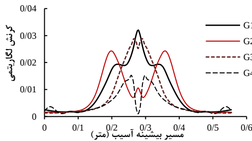
شکل ۱۷- کرنش در مسیر بیشینه آسیب
