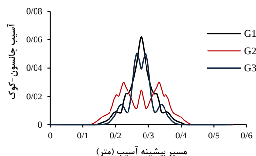
شکل ۱۹- آسیب وارده به مخازن براساس معیار جانسون-کوک
