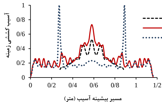
شکل ۹- آسیب کششی وارده به زمینه براساس معیار هاشین
