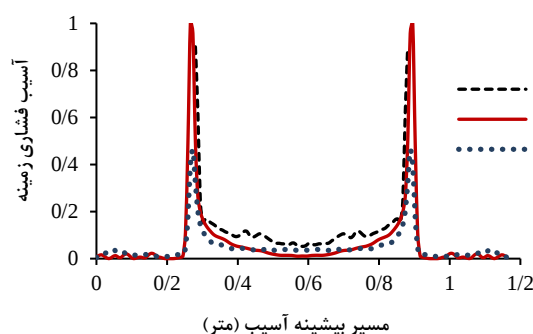
شکل ۱۵- آسیب فشاری وارده به زمینه براساس معیار هاشین
