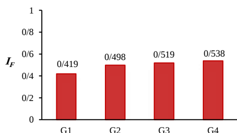
شکل ۲- مقدار بحرانی‌ترین شاخص شکست سای هیل ( I_F )
