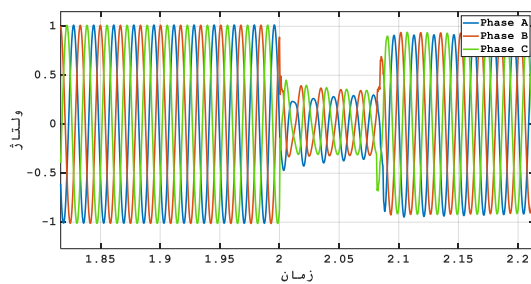
شکل ۸- ولتاژ در باس ۷
