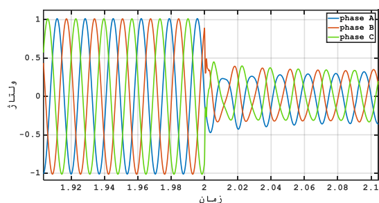
شکل ۱۲ - ولتاژ در باس ۷
