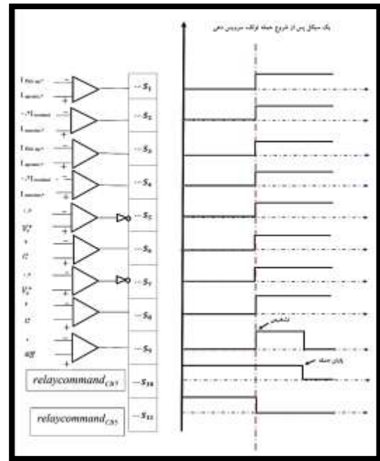
شکل ۳۰- بردار سیگنال منطقی خروجی در حمله توقف سرویس دهی
