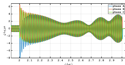
شکل ۲۷ - جریان خط از سمت باس ۷
