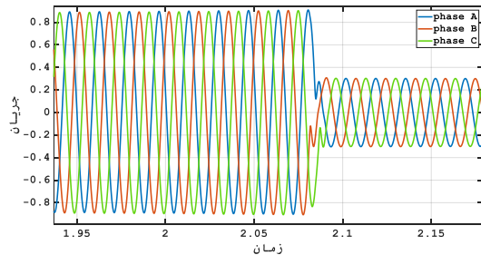
شکل ۱۷- جریان خط از سمت باس ۵
