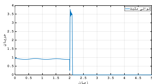
شکل ۱۴ - توالی مثبت جریان باس ۵
