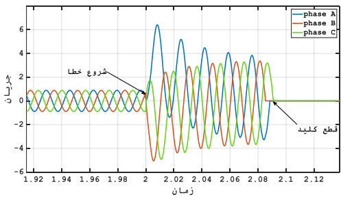
شکل ۷- جریان خط از سمت باس ۵
