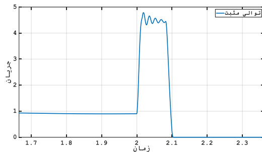
شکل ۱۸- توالی مثبت جریان باس ۷
