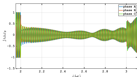
شکل ۲۳ - ولتاژ در باس ۷
