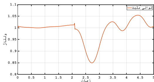
شکل ۲۰- توالی مثبت ولتاژ باس ۷
