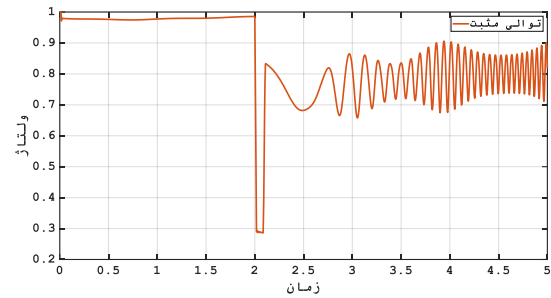
شکل ۱۶- توالی مثبت ولتاژ باس ۵
