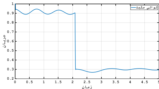
شکل ۱۹- توالی مثبت جریان باس ۵
