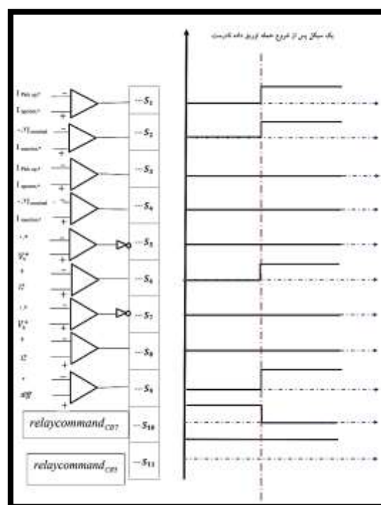
شکل ۲۹- بردار سیگنال منطقی خروجی در حمله تزریق داده نادرست
