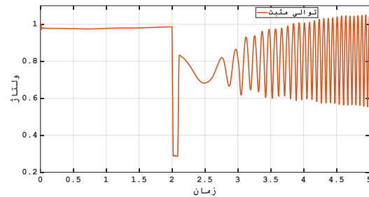
شکل ۲۶ - توالی مثبت ولتاژ باس ۵
