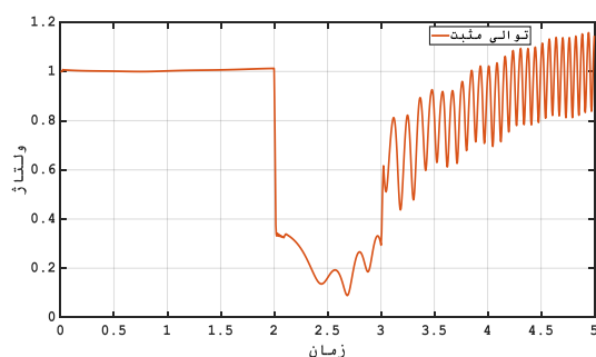
شکل ۲۵ - توالی مثبت ولتاژ باس ۷
