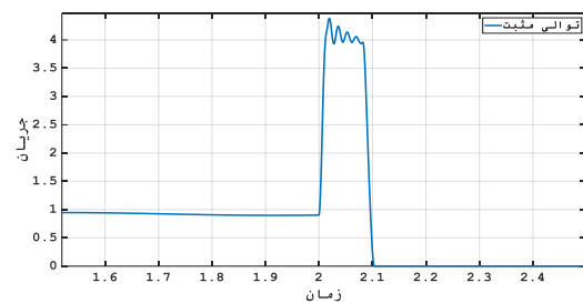
شکل ۹- والی مثبت جریان باس ۷
