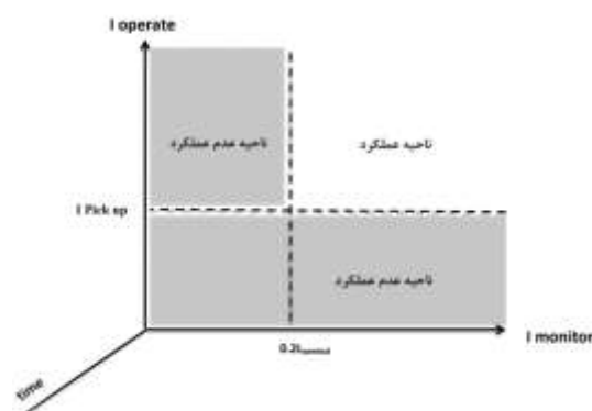
شکل ۱- مشخصه پیشنهادی رله اضافه جریان
