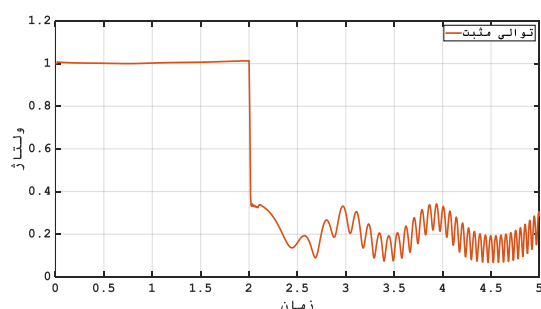
شکل ۱۵ - توالی مثبت ولتاژ باس ۷
