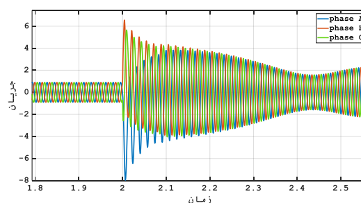
شکل ۱۶ - جریان خط از سمت باس ۷
