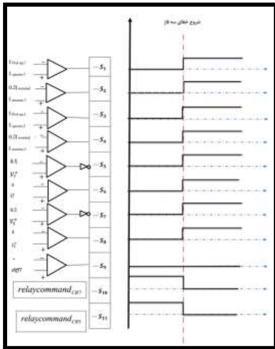
شکل ۲۷- بردار سیگنال منطقی خروجی در خطای سه فاز
