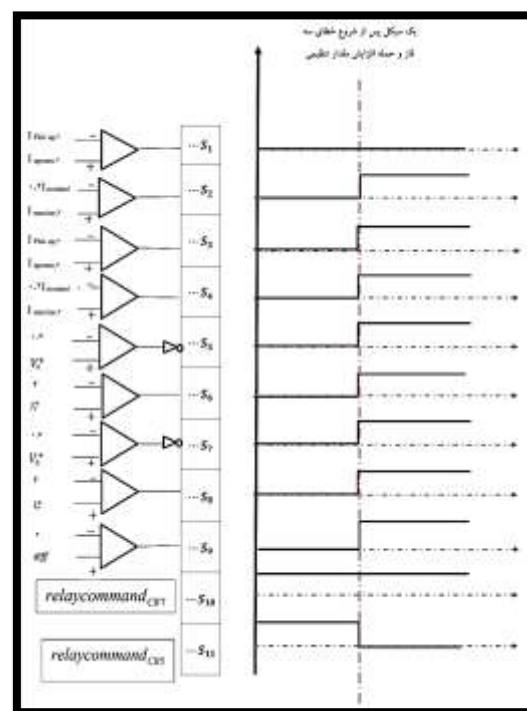
شکل ۲۸- بردار سیگنال منطقی خروجی در حمله افزایش مقدار تنظیمی
