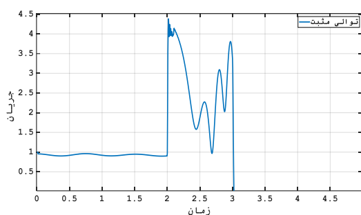
شکل ۲۴ - توالی مثبت جریان باس ۷
