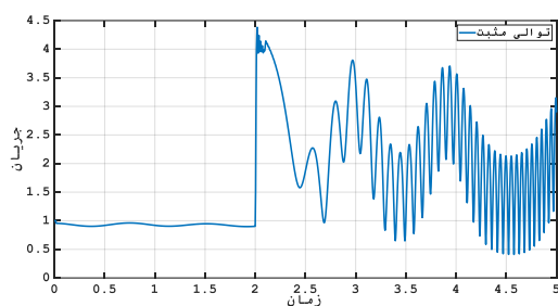
شکل ۱۳ - توالی مثبت جریان باس ۷
