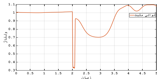
شکل ۱۰- توالی مثبت ولتاژ باس ۷
