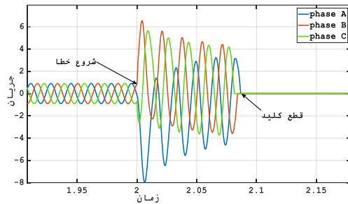
شکل ۶- جریان خط از سمت باس ۷
